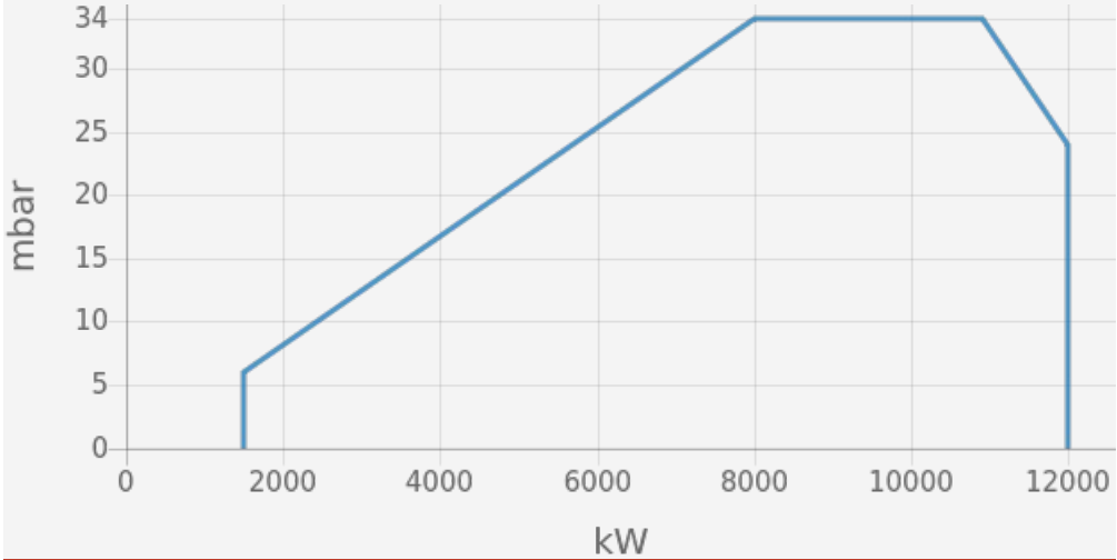
工作曲线
