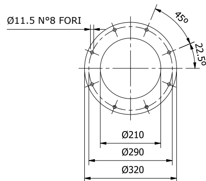
DETTAGLIO FLANGIA DI FISSAGGIO
