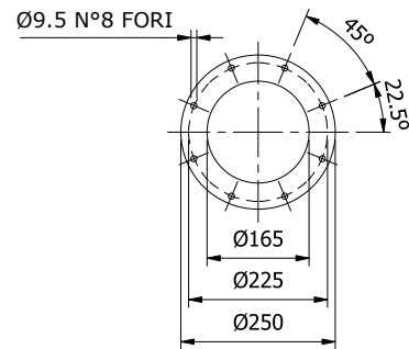
DETTAGLIO FLANGIA DI FISSAGGIO
