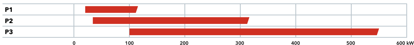
PISTOLENBRENNER / GAS 17 / 500 kW
