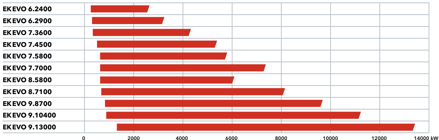
/ GAS BAUREIHE 340 / 13500 kW
