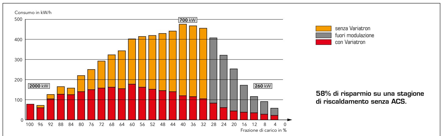
Fig. 2 - Distribuzione dei consumi elettrici di un bruciatore durante l'intera stagione di riscaldamento.
